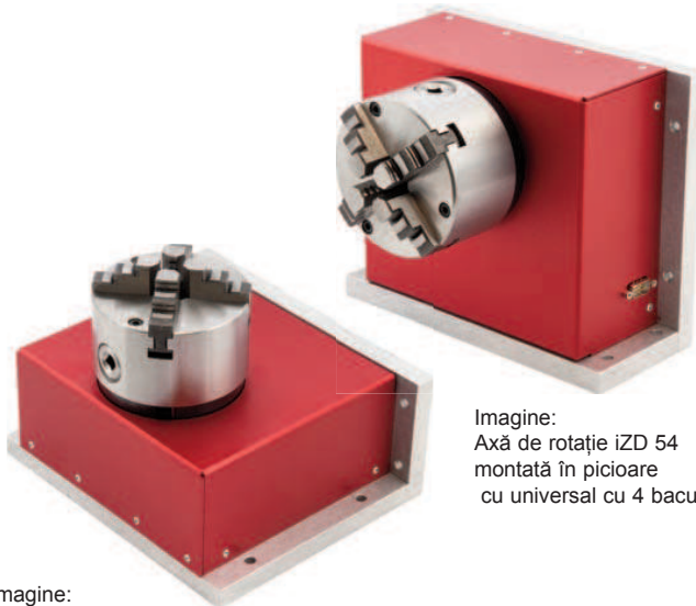
Imagine: Axă de rotație iZD 54 montată plan cu universal cu 4 bacuri
