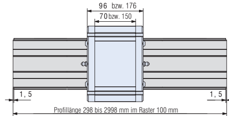
LFS-8-4 cu cărucior LW 7
