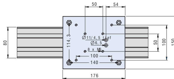
LFS-8-4 cu cărucior LW 7
